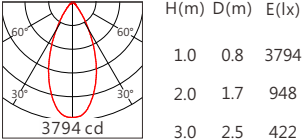
OSRAM SSL80 45° 3000K
