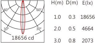
OSRAM SSL80 15° 4000K
