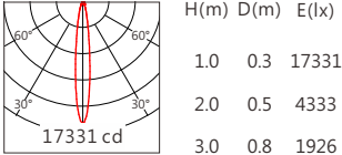
OSRAM SSL80 15° 3000K
